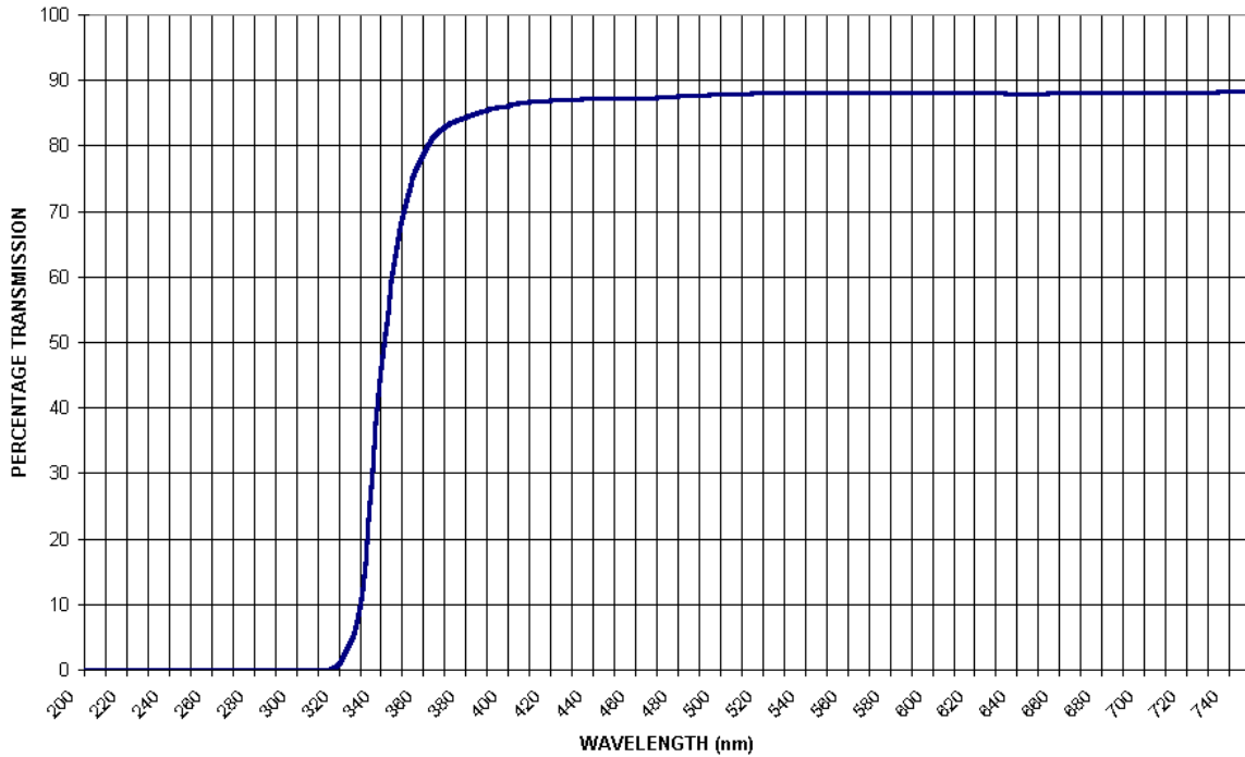
HOYA UV-34 (200 - 750 nm)
